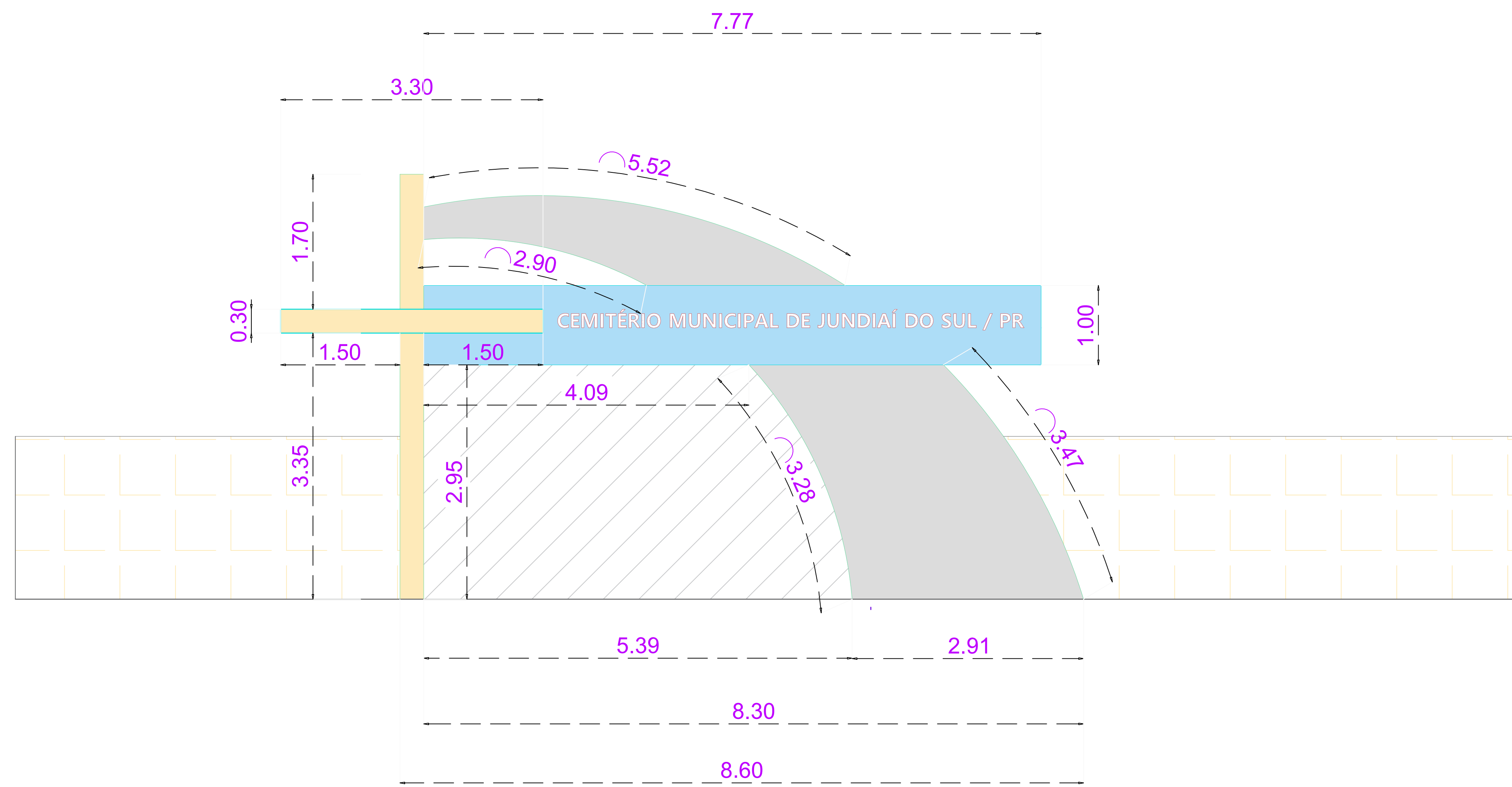
ELEVAÇÃO FRONTAL - ESCALA 1/50
