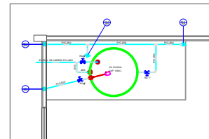
HIDRÁULICO - ABASTECIMENTO ESCALA: 1:50
