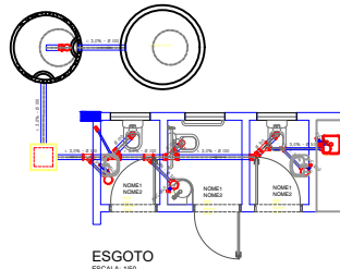
ESGOTO ESCALA: 1:50
