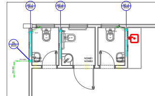
HIDRÁULICO ESCALA: 1:50
