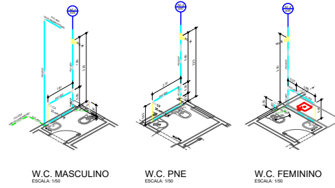
W.C. MASCULINO ESCALA: 1:50
