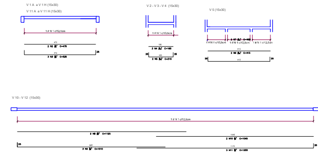
FORMAS VIGAS BALBRAME Escala 1 - 75
