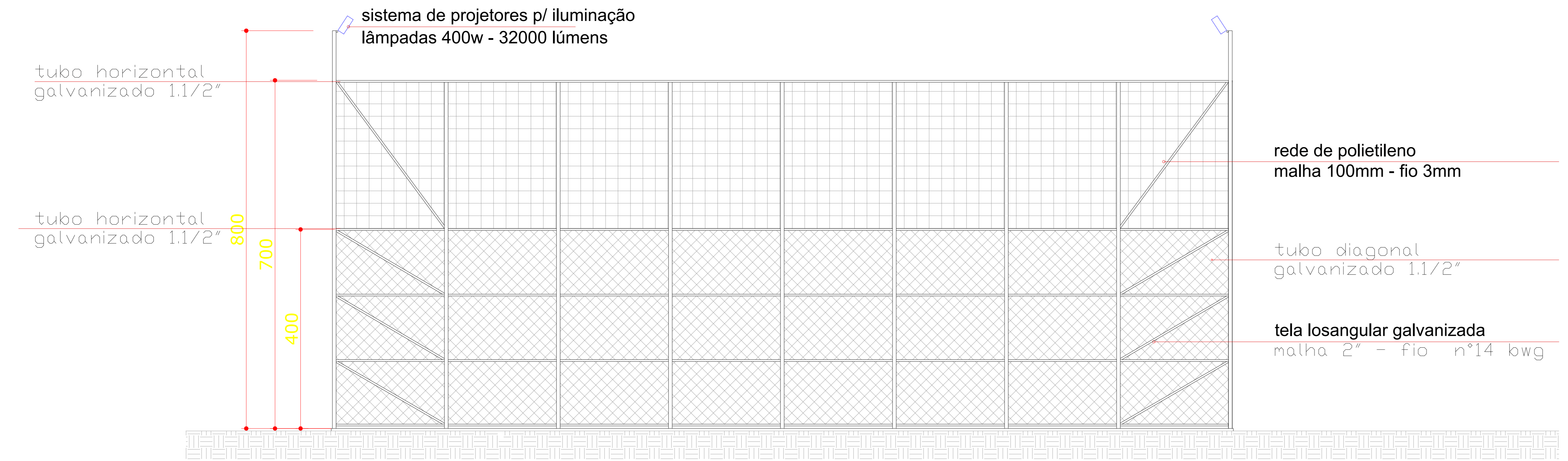
ELEVAÇÃO FRONTAL escala 1:100
